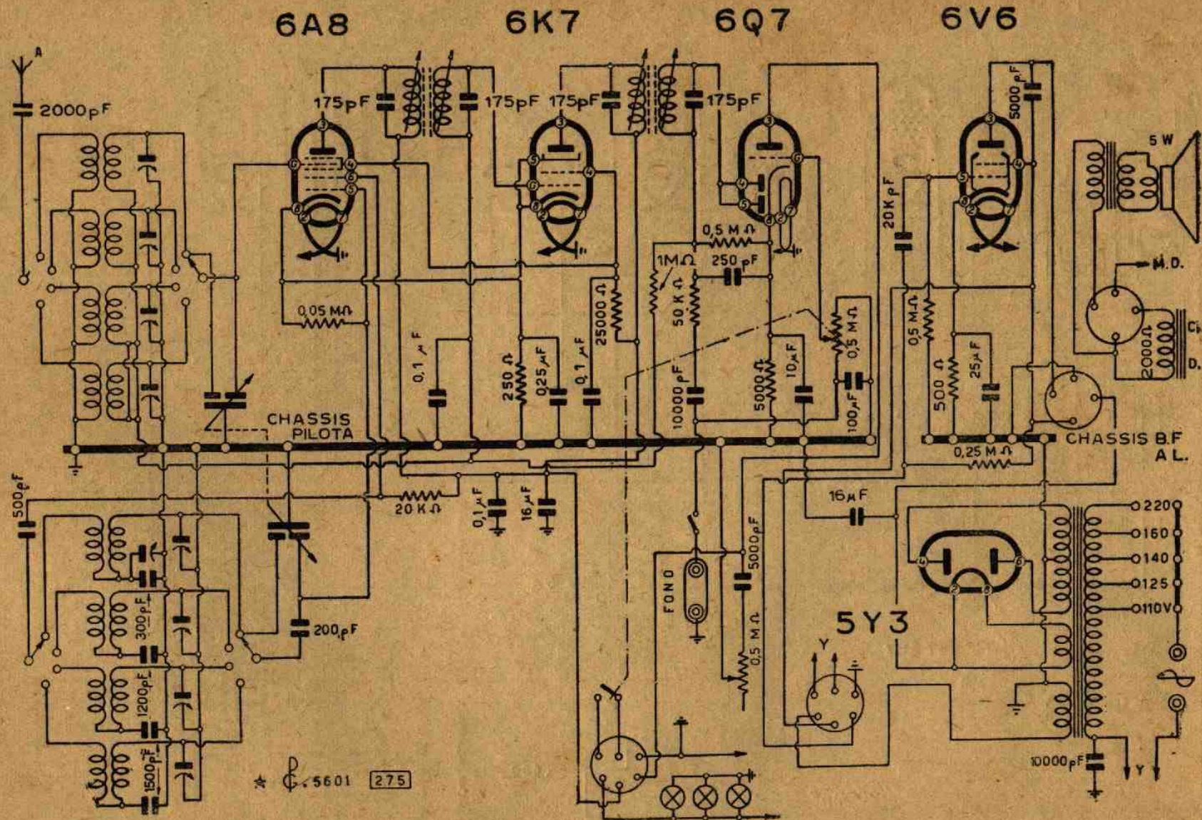
Lo schema elettrico del mod. 542
